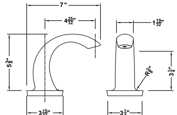
Faucet Stem SSFS01
